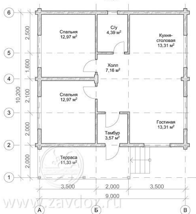
План
